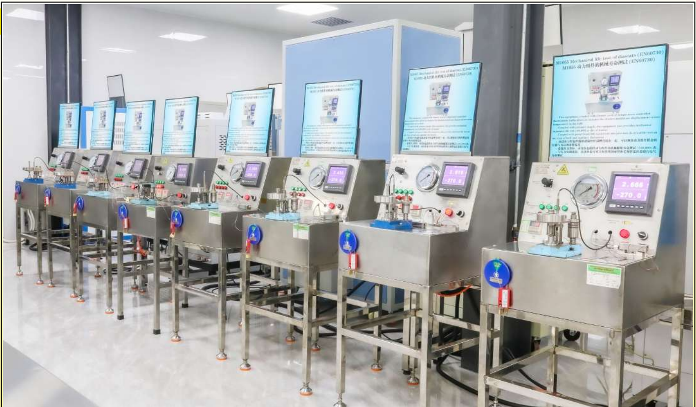
Un set di apparecchiature automatiche per test di durata meccanica diastat. Ogni apparecchiatura ha un registratore dati dei parametri di test e del numero di cicli (Laboratorio Ultimateheat).
